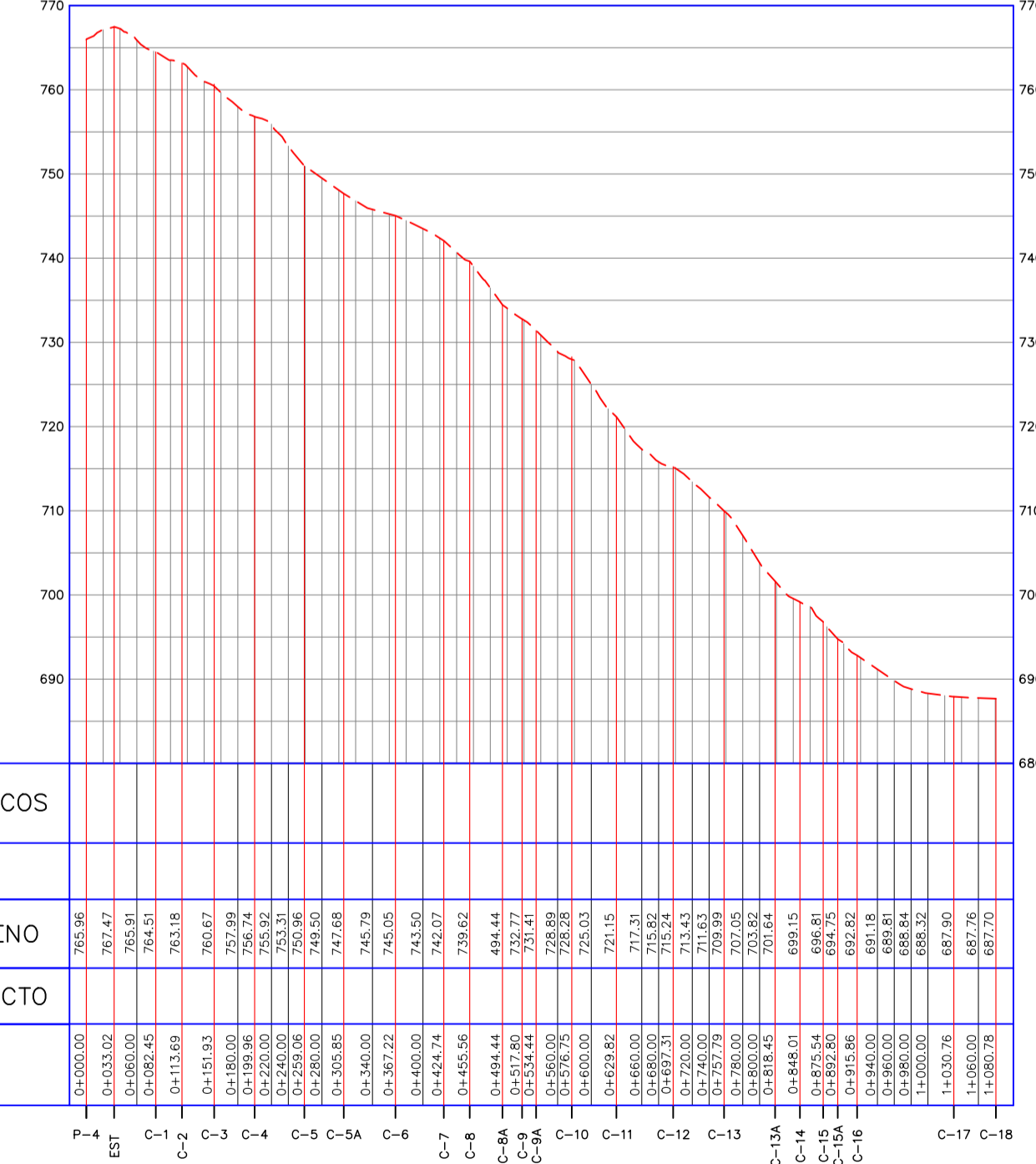
PERFIL Escala H = 1:7500 V = 1:75000
